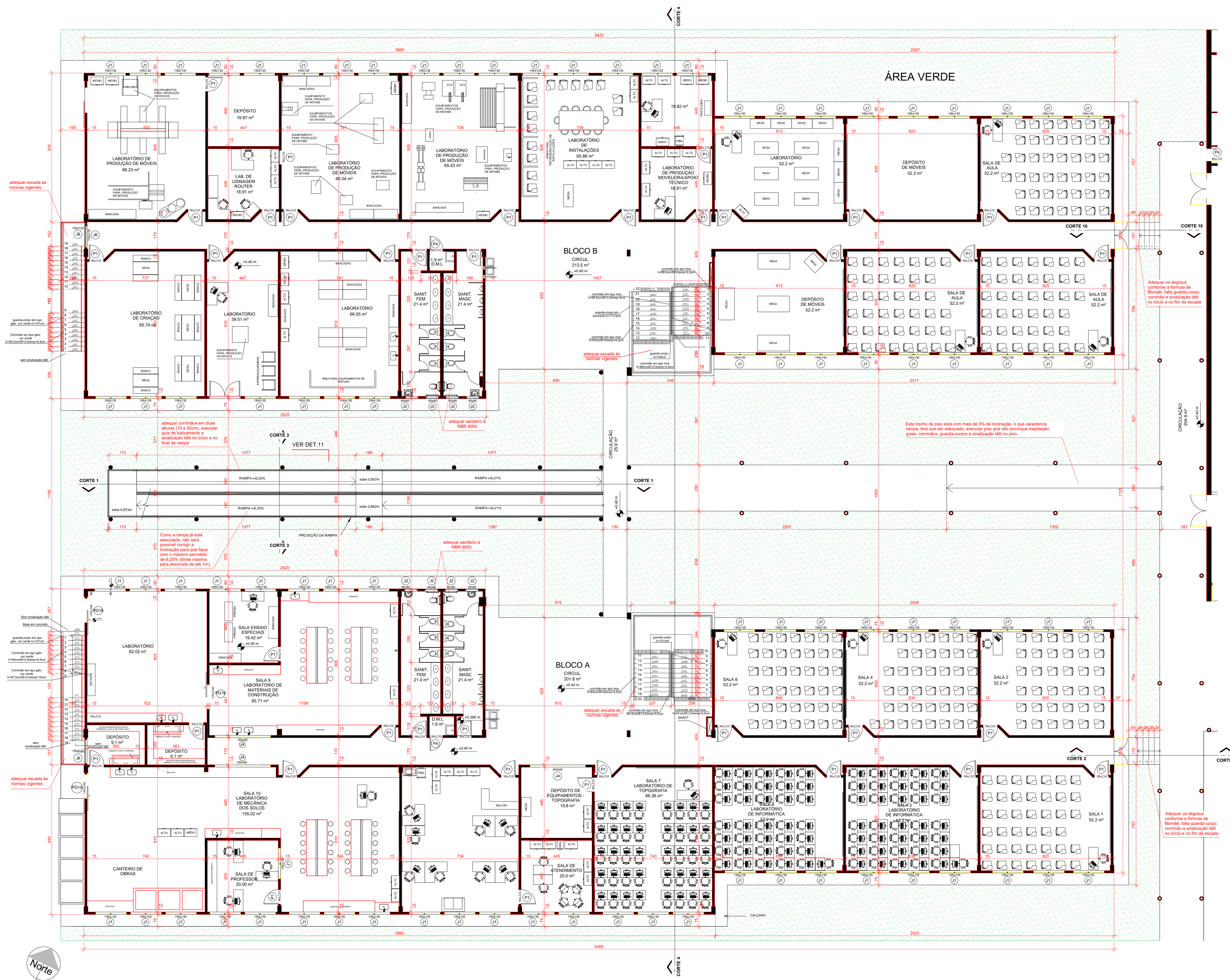
DIAGNÓSTICO/SITUAÇÃO ATUAL - TÉRREO 1 : 100
